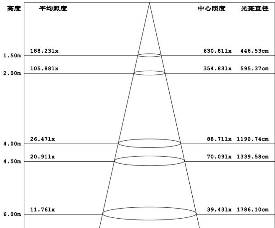
光束角:112.2度
