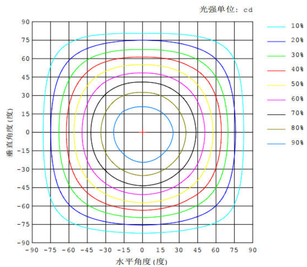
光束角:112.2度
